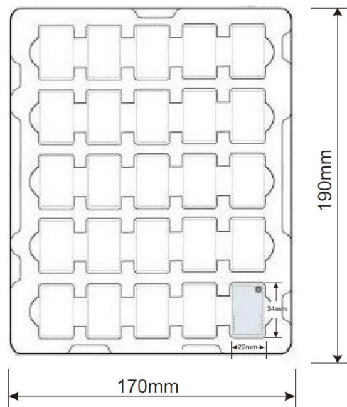
正面图
