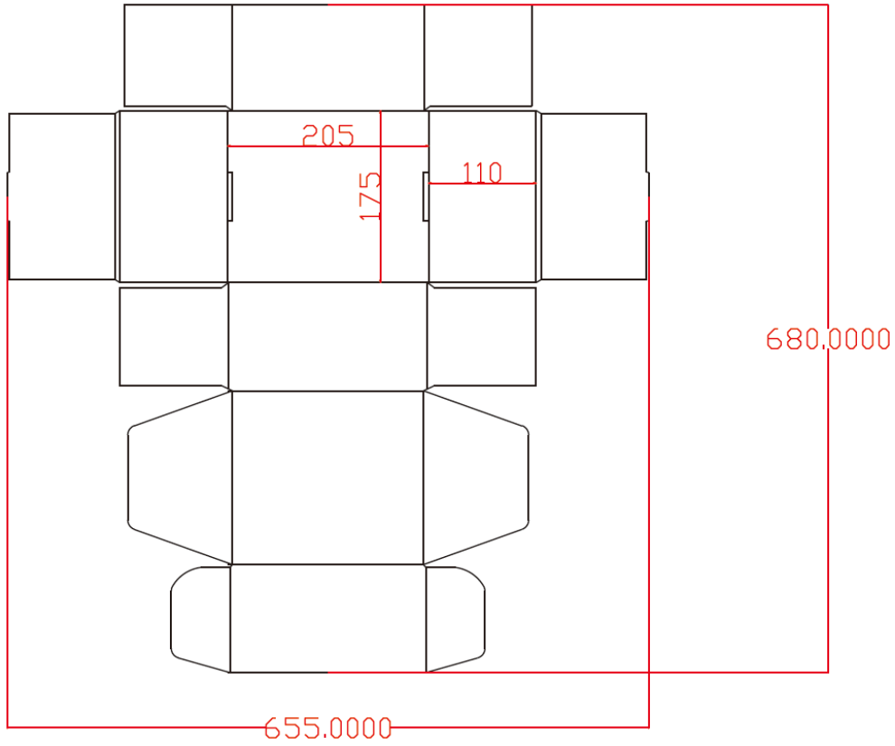
正面图
