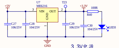
3.3V电源
