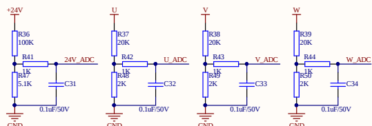
电压采样电路
